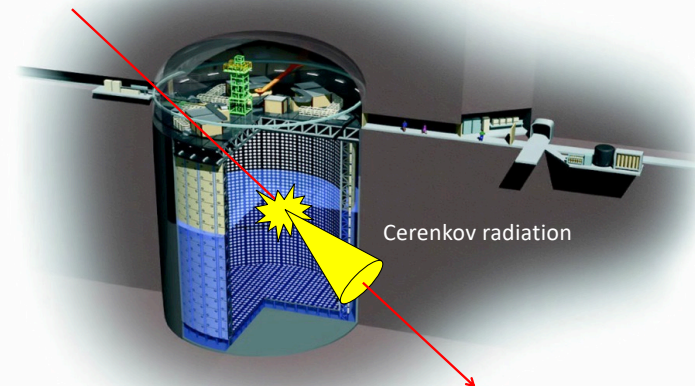
Super-Kamiokande
